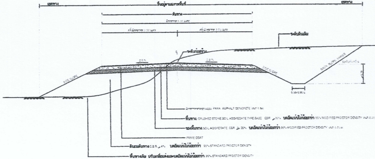
รูปตัดแสดงโครงสร้างถนน คัดดิน ดินถม และคุณสมบัติวัสดุ ช่วง STA (0+000 - 1+180)
